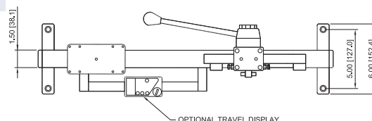
TSA750H
